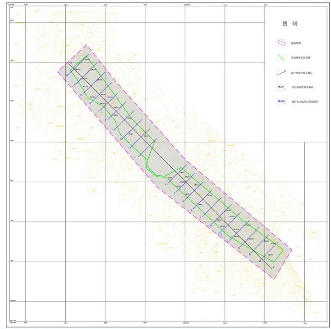
湖北省广水市六猪咀-刘家河矿区建筑用灰岩矿勘查工作预布置图 1: 5000
